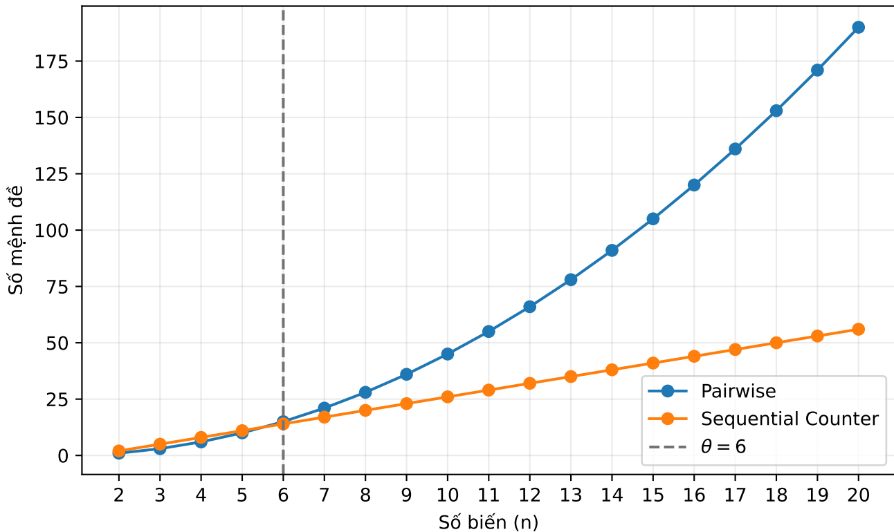
Số mệnh đề mã hóa AMO theo lý thuyết
