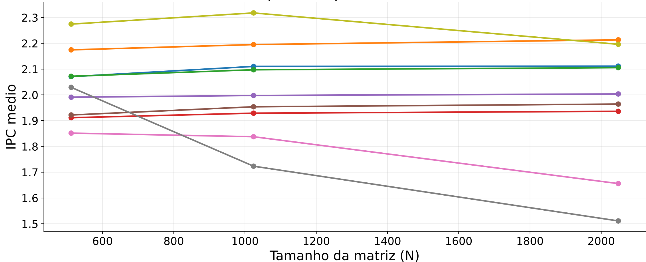
Instrucoes por ciclo por tamanho da matriz
