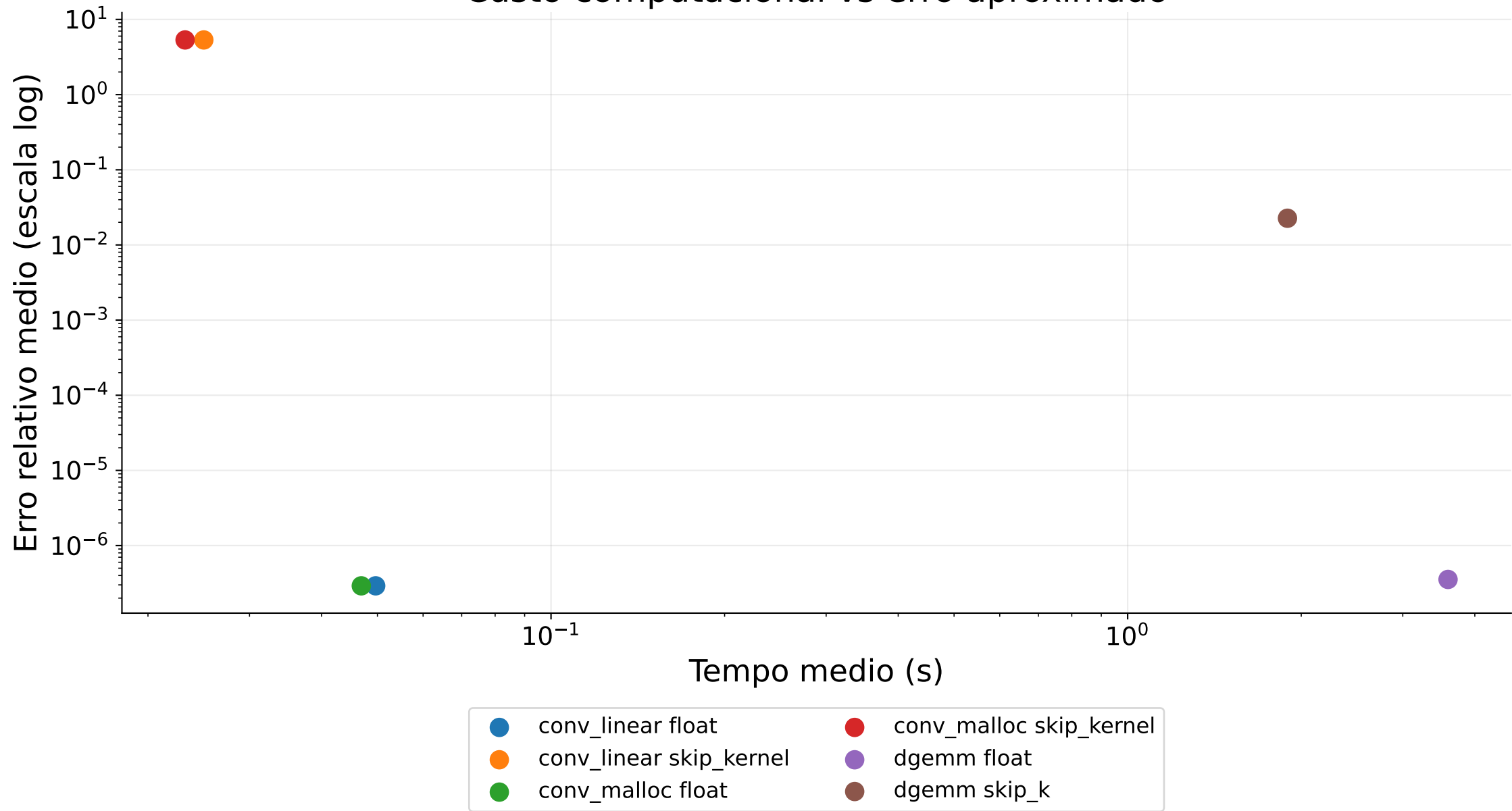
Custo computacional vs erro aproximado
