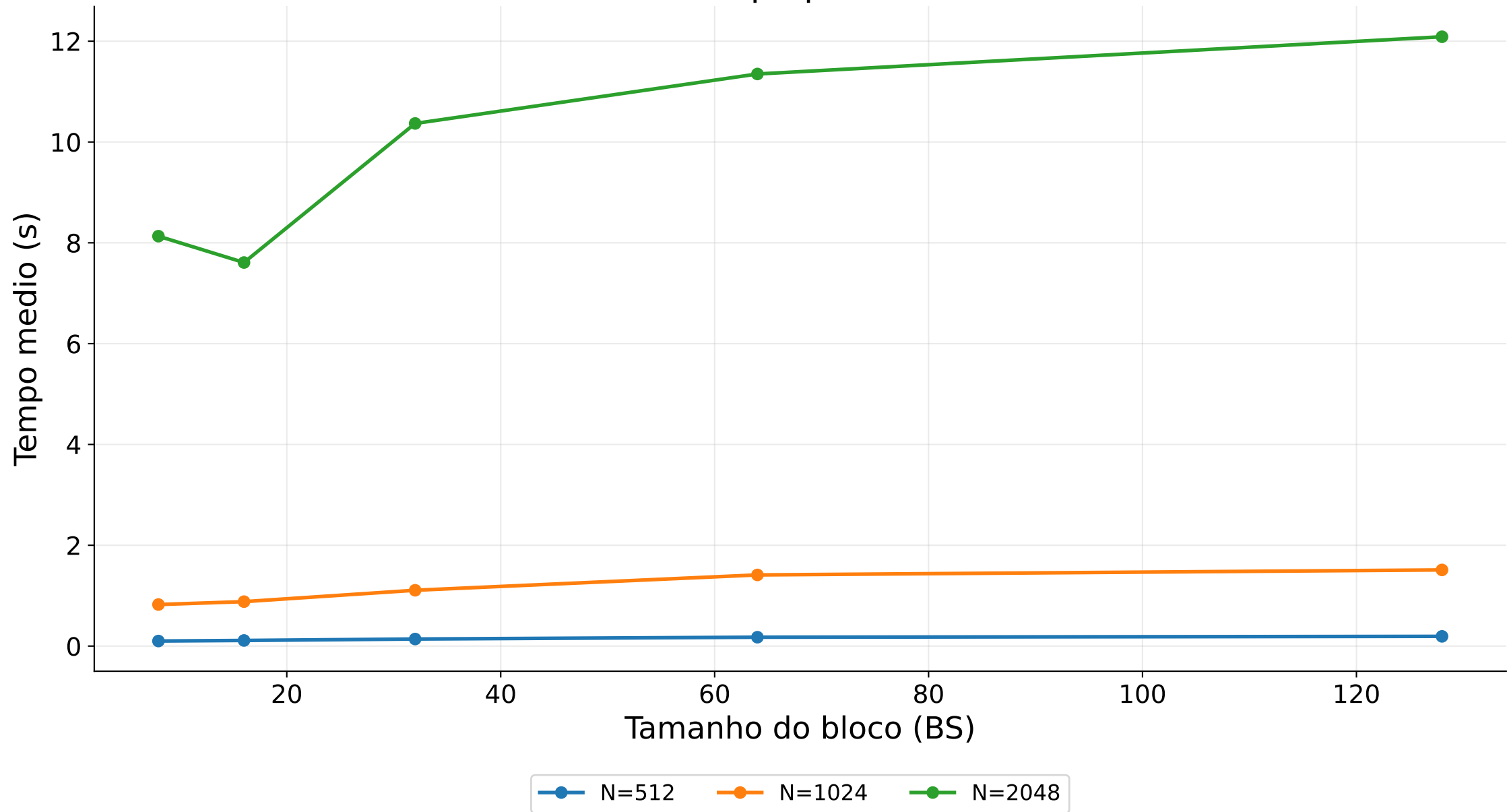
DGEMM exato: tempo por tamanho de bloco
