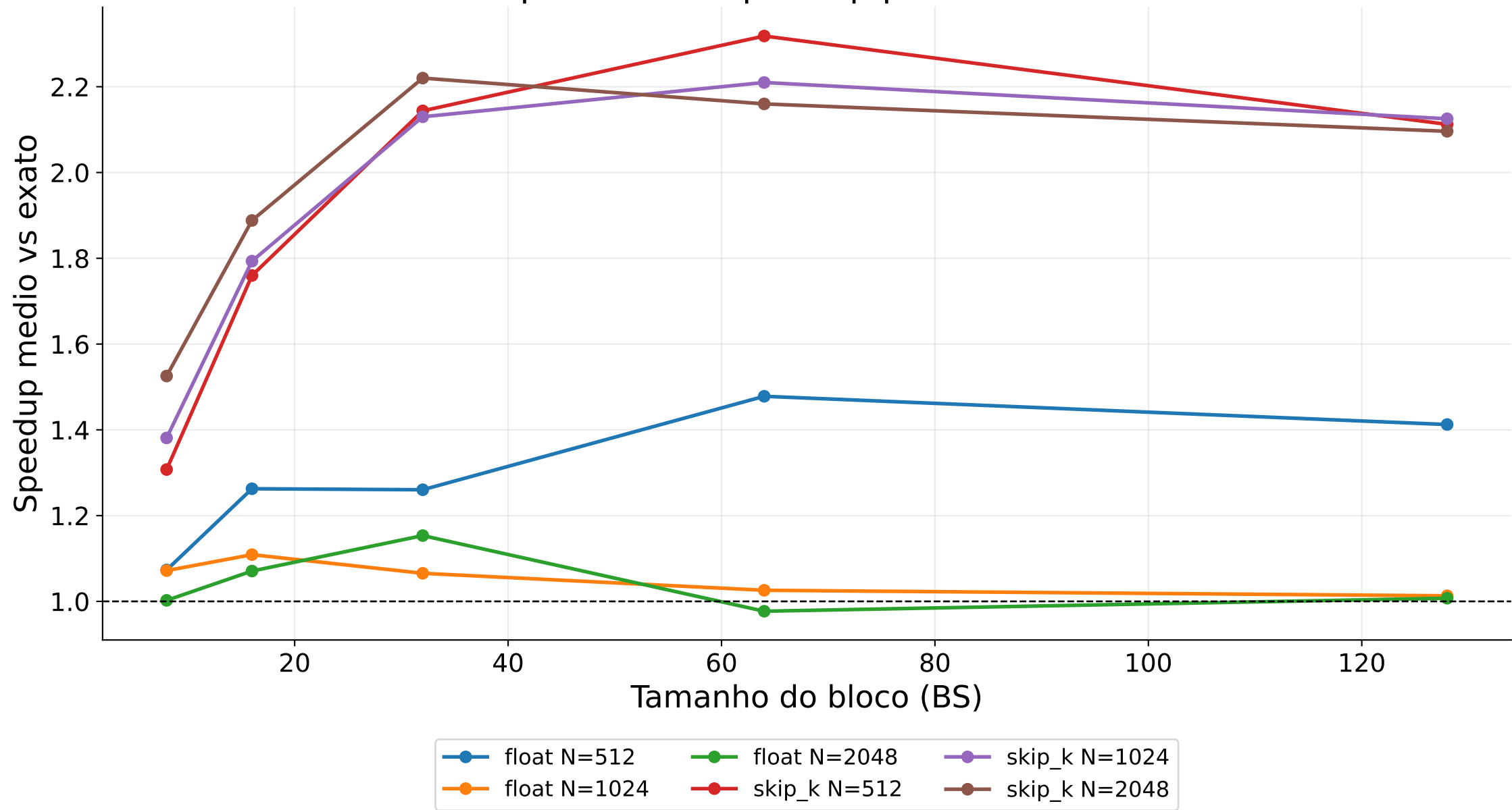
DGEMM aproximado: speedup por tamanho de bloco
