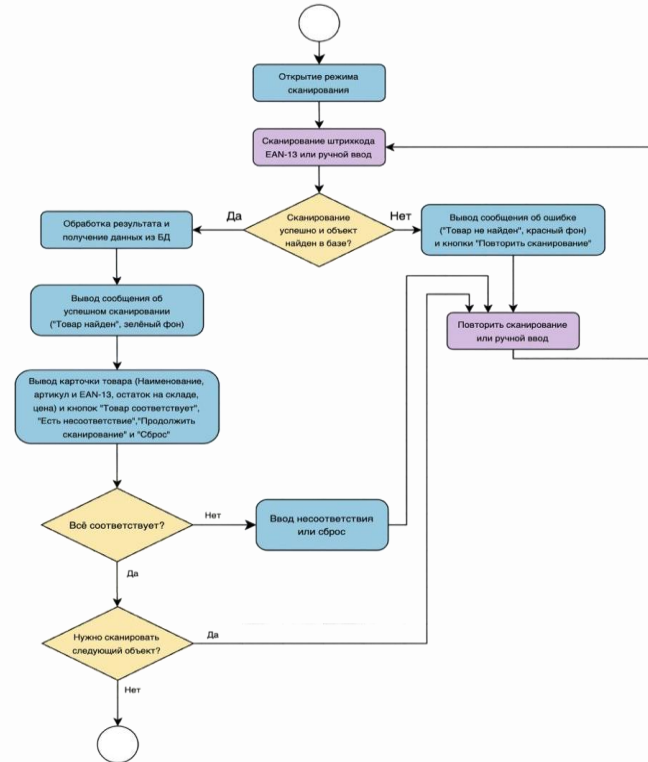
Блок-схема алгоритма сканирования
