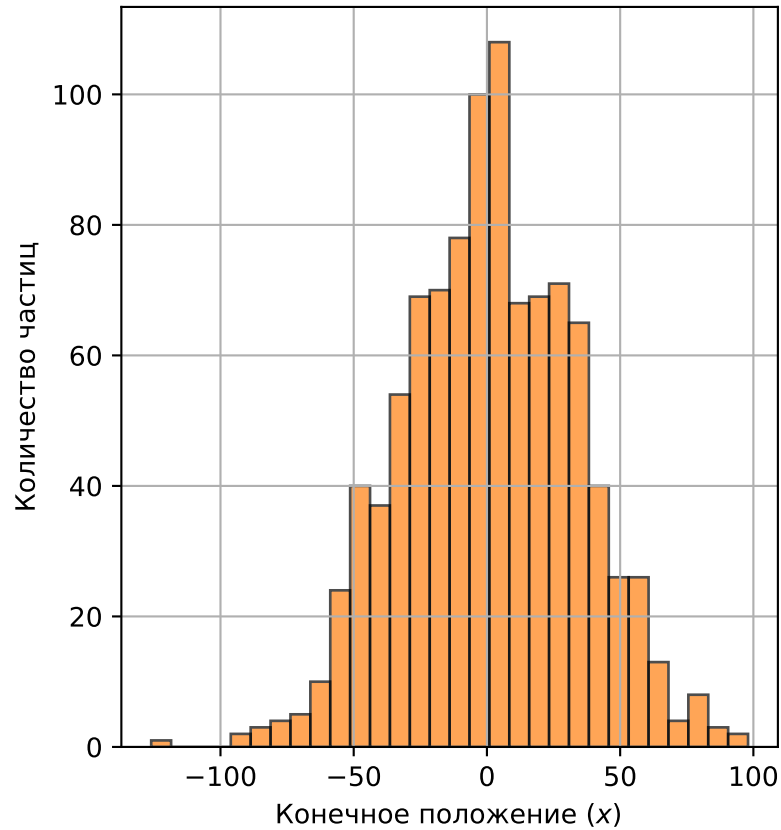
Гистограмма положений после 1000 шагов
