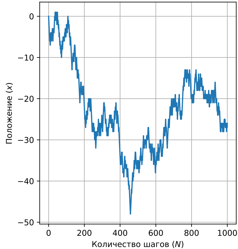
Траектория одной частицы x(N)
