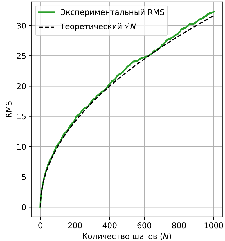
Зависимость RMS от шагов N
