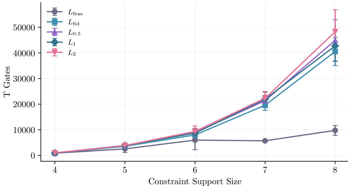
Study A: FTQC Gadget T Gates
