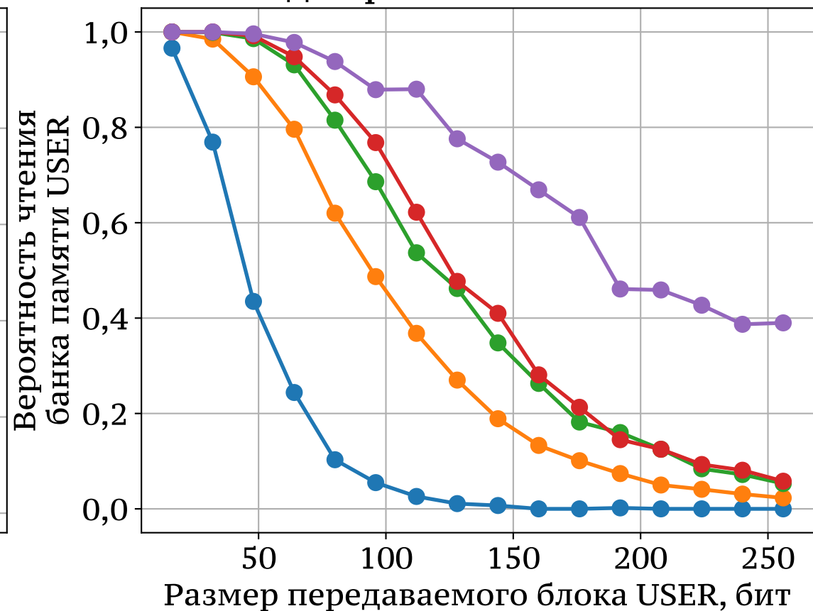
Вероятность от длины банка USER для разных Tari и M
