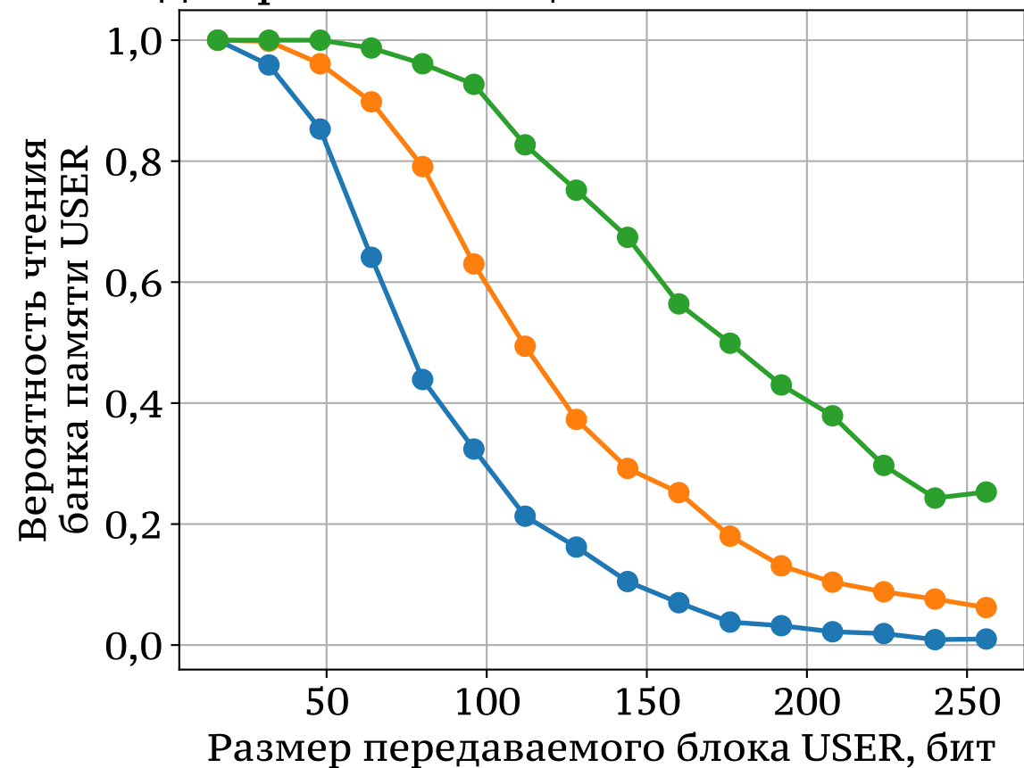
Вероятность от длины банка USER для разных мощностей считывателя
