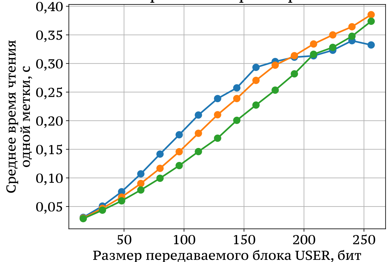
Зависимость времени от размера блока памяти
