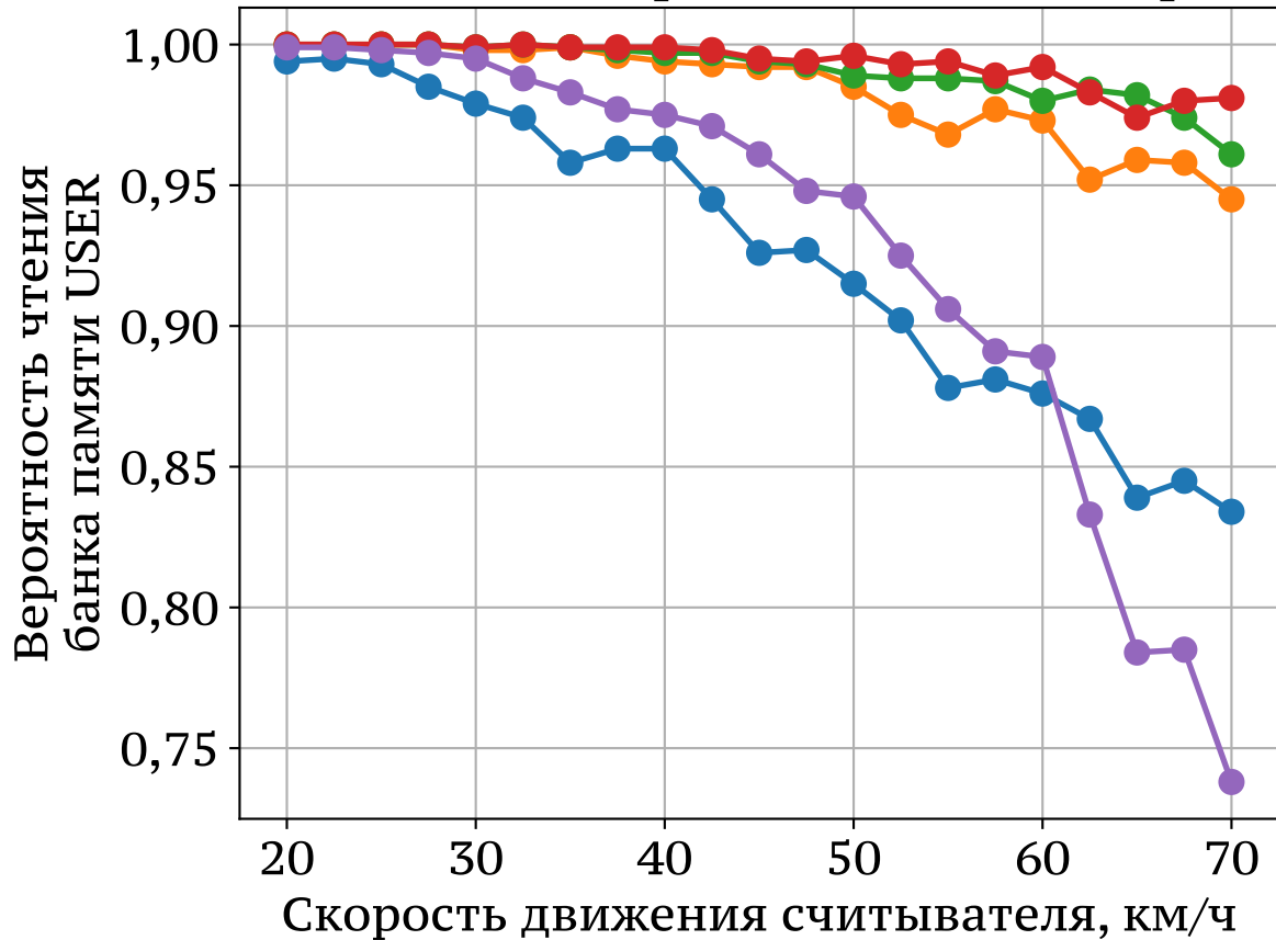
Зависимость вероятности от скорости
