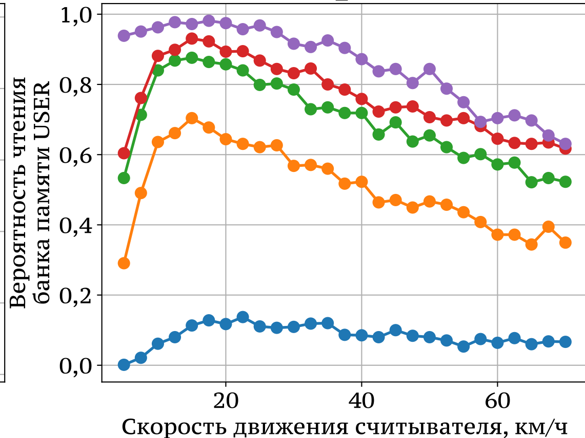
Зависимость вероятности от скорости для reader_offset = 1.0
