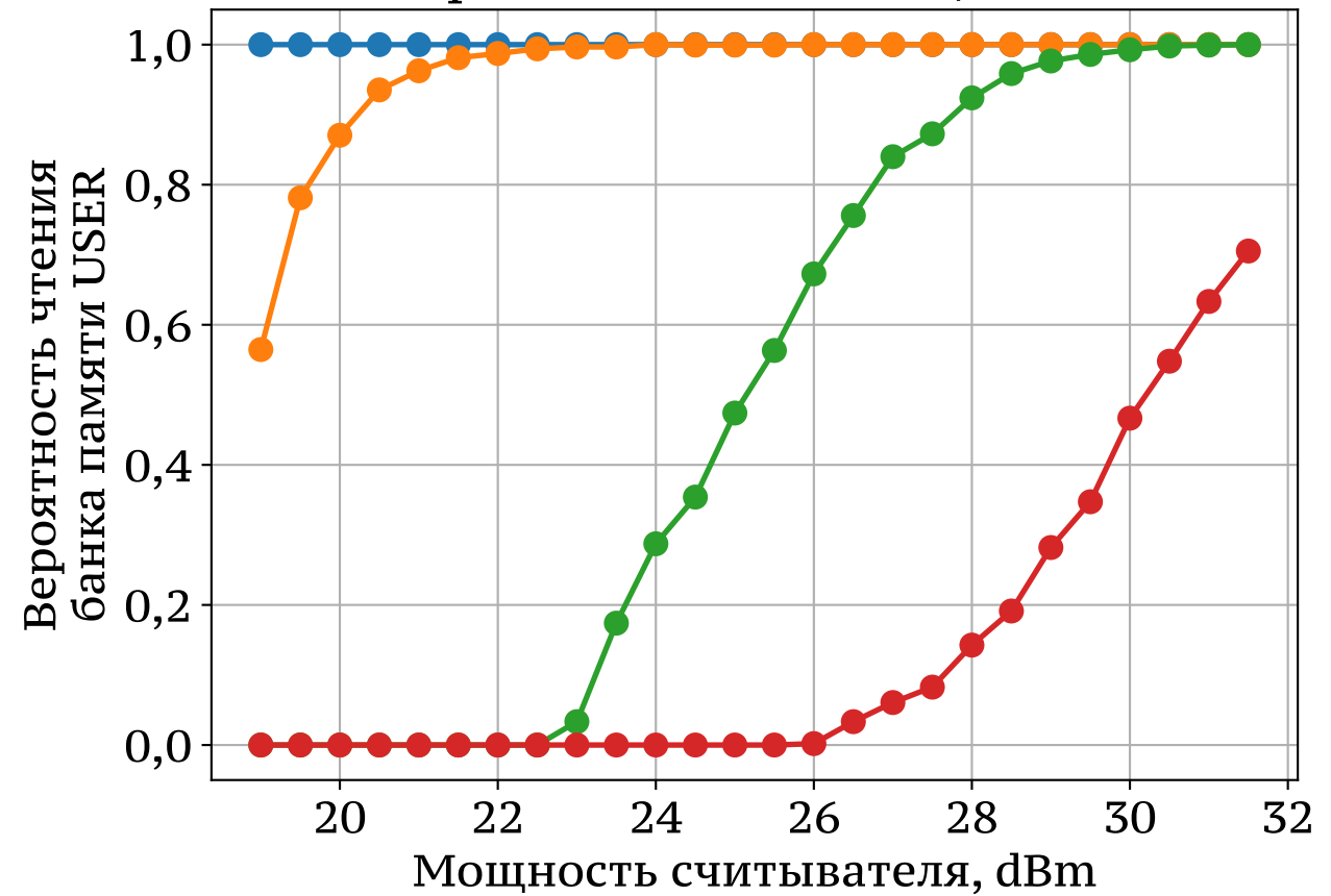
Зависимость вероятности от мощности считывателя
