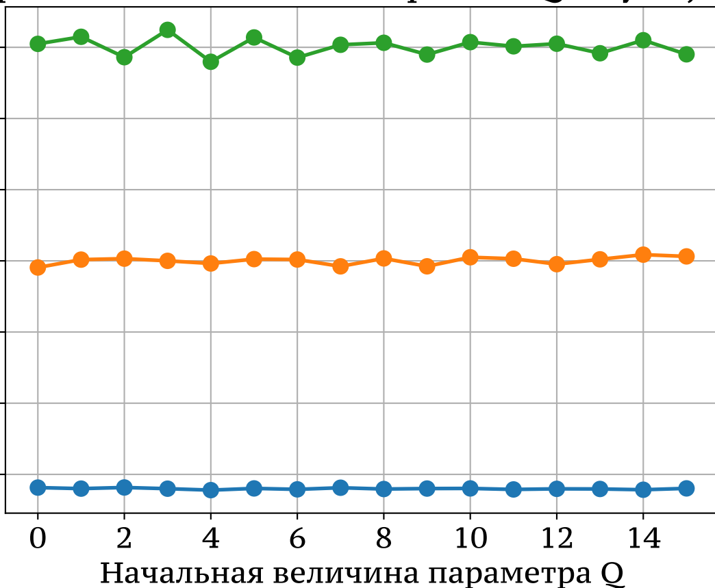
Зависимость времени от стартового Q при использовании алгоритма QueryAdjust
