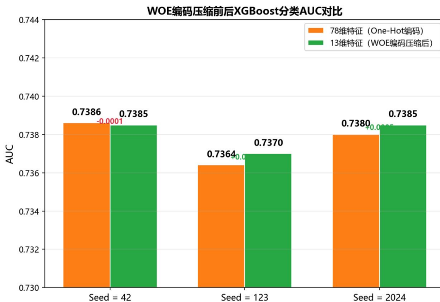
图 2 WOE 编码压缩前后分类模型的 AUC 对比图
