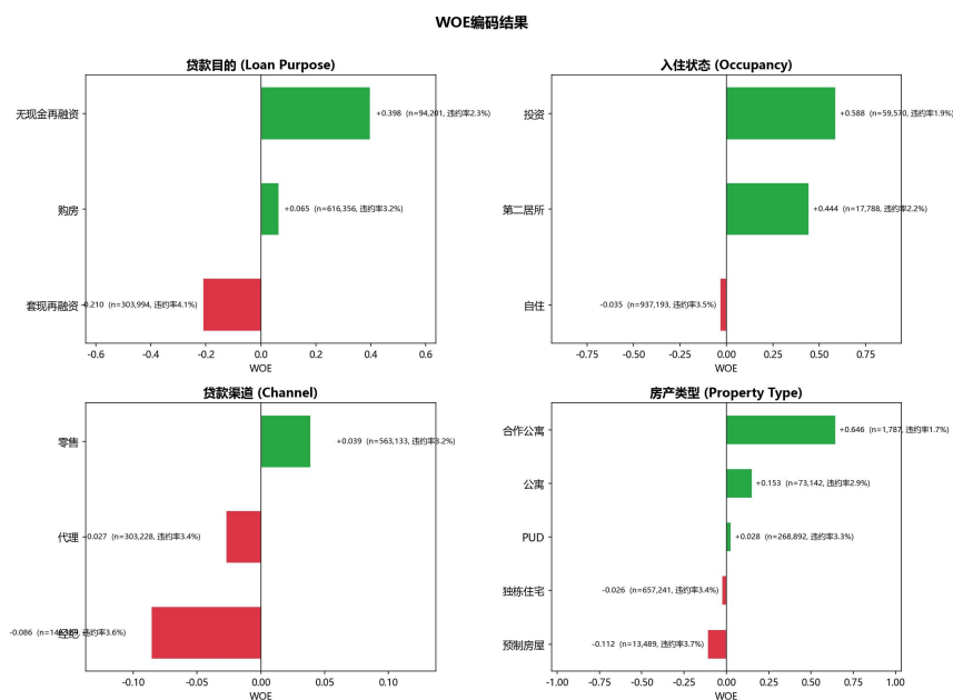
图 1 WOE 编码结果
