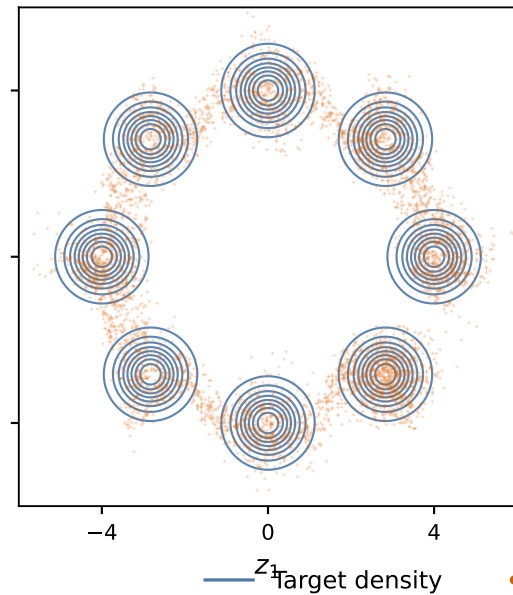
RealNVP-4 seed 46 · ELBO -0.348 · SW 2 0.380
