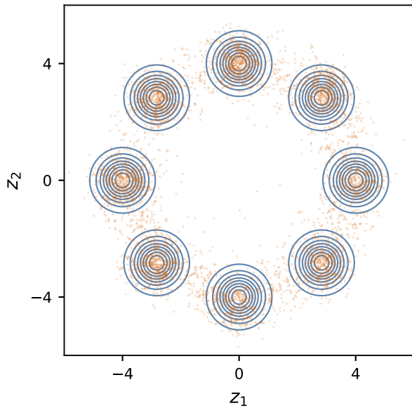
DIVI seed 45 · ELBO -0.167 · SW 2 0.214
