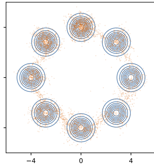
RealNVP-8 seed 42 · ELBO -0.285 · SW 2 0.556
