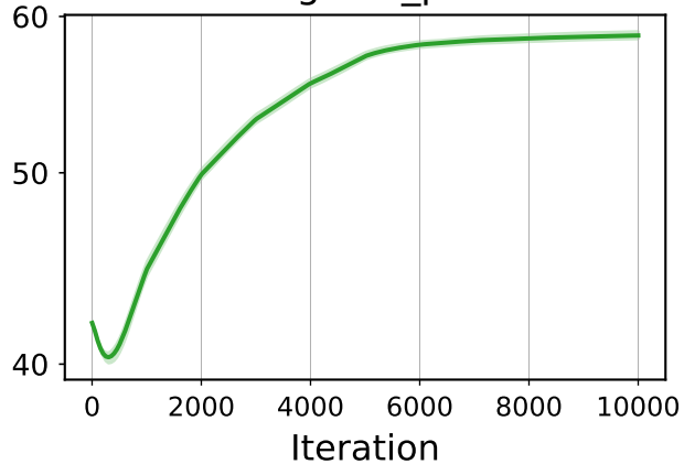
Langevin_post
