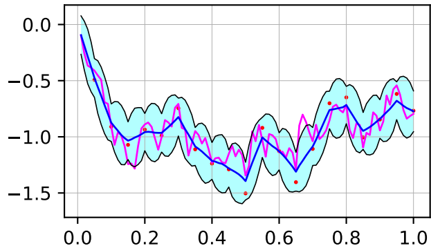
DSIVI
