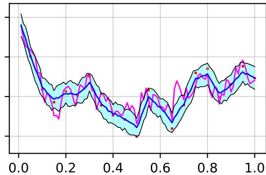
KSIVI
