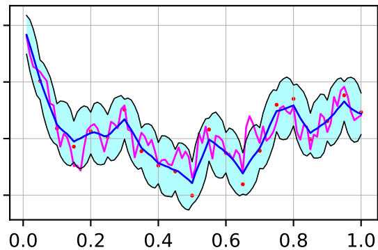
AISIVI
