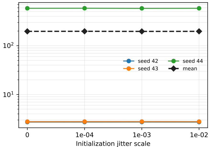
Score R-hat p95
