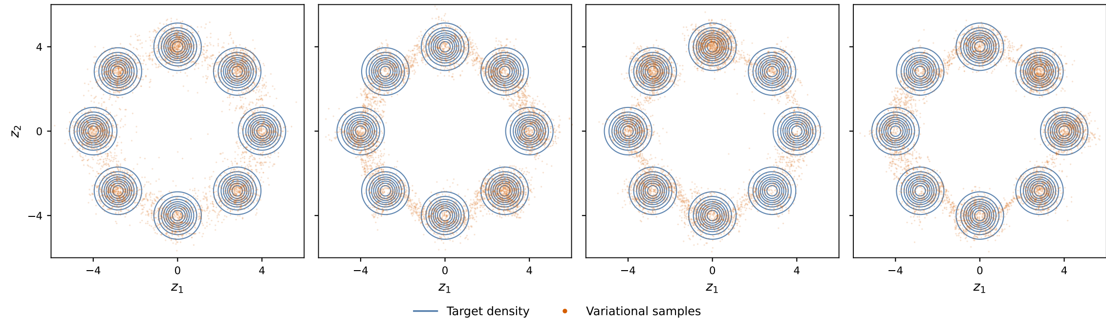
DIVI seed 45 · ELBO -0.167 · SW 2 0.214
