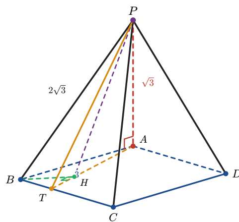
(图 2) 四棱锥 P-ABCD 结构图 ( PA \perp 底面, BH \perp AT )
