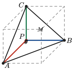
第6题 三棱锥补成长方体： PA 、 PB 、 PC 沿三条坐标轴且两两垂直，等于体对角线的一半
