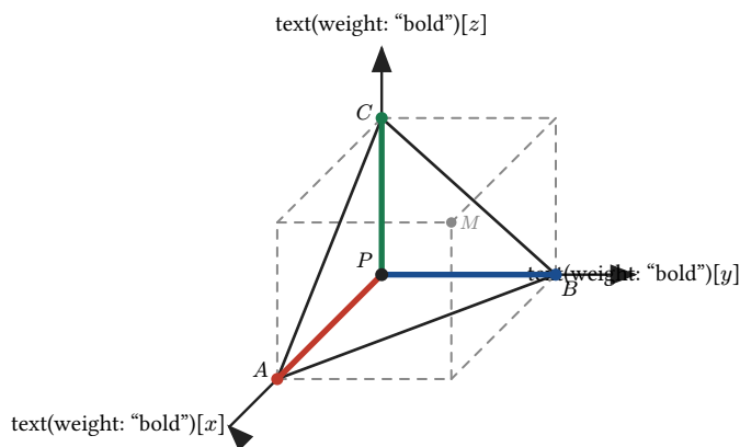
第6题 三棱锥补成长方体：PA、PB、PC沿三条坐标轴且两两垂直，等于体对角线的一半
