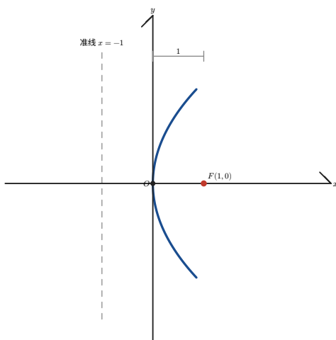
第 1 题 2p = 4 \Rightarrow p = 2 ，焦点 F(1, 0) ，准线 x = -1
