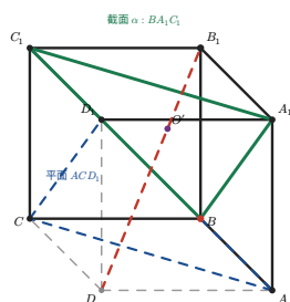
第 11 题 左: 正方体轴测投影与内切球截面平面 \alpha (平行于 ACD_1 ); 右: 截面 \alpha 内几何解析
