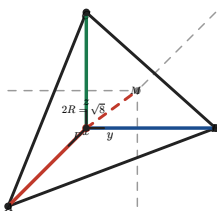
第6题 补成长方体：PA、PB、PC 沿三坐标轴，两两垂直；P 与体对角顶点 M 连成外接球直径
