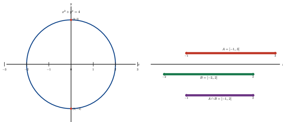
第 2 题 A = [-1, 3] 与 B = [-2, 2] 取交得 [-1, 2]
