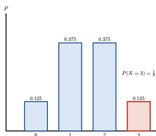
第 5 题 X \sim B(3, \frac{1}{2}) , 所求为“三件全为次品”之外的全部情形
