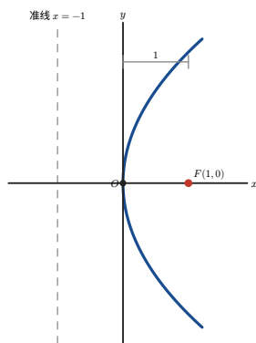
第 1 题 2p = 4 \Rightarrow p = 2 ，焦点 (1, 0) ，准线 x = -1
