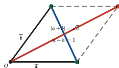
第 3 题 平行四边形: 红色为 |a + b| = \sqrt{3} , 蓝色为 |a - b| = 1 对应的对角线
