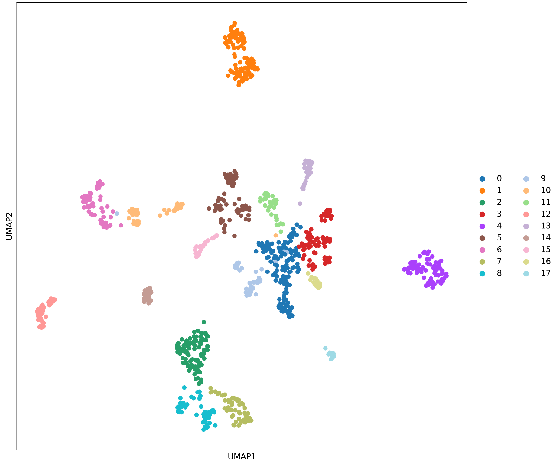
Cell Clusters (Leiden)
