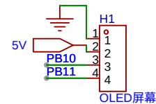
OLED屏幕
