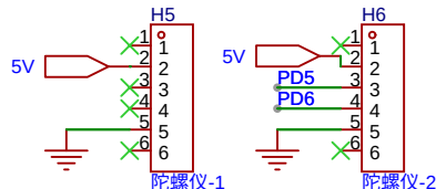
陀螺仪
