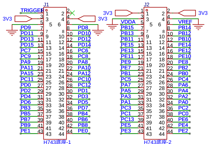
H743底座
