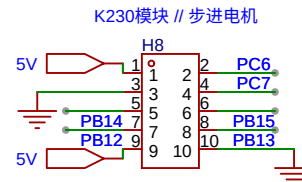
集成模块
