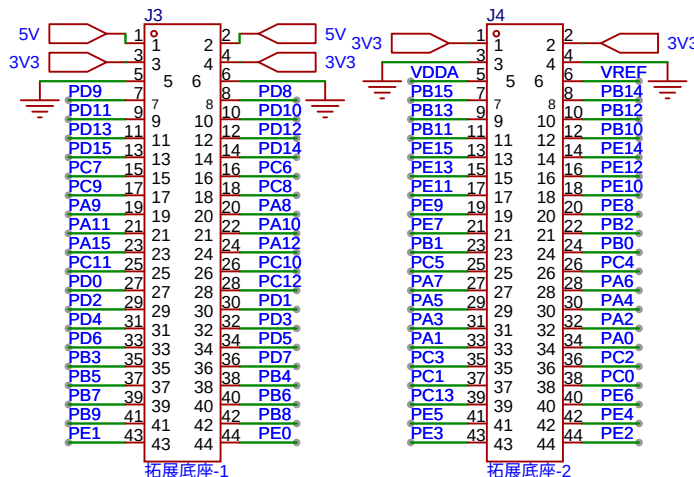
拓展底座
