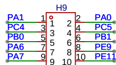
电机/编码器
