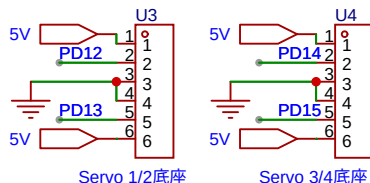
舵机
