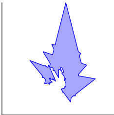
Iterata 3
