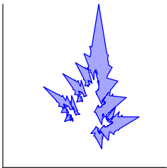
Iterata 5
