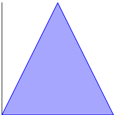
Seme dell'algoritmo
