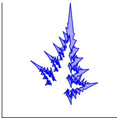
Iterata 7
