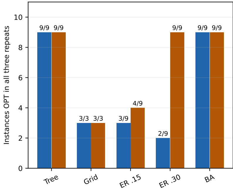
L(1,1)
