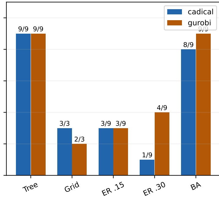
L(3,2)
