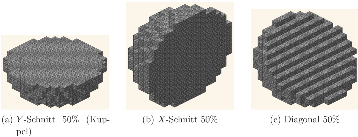
Abbildung 4: Drei Schnitte durch dieselbe Kugel D = 16 , jeder erhält 50% des Volumens. Der Y -Schnitt erzeugt die klassische Kuppel V_{\text{Kuppel}} = \frac{2}{3}\pi r^3 ; der diagonale Schnitt legt die Hypotenuse x + y = k frei, die für diese Schnittebene charakteristisch ist.
