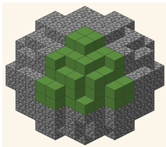
Figure 7: D = 10 の球で、正の八分象限 (+x, +y, +z) を緑で強調表示。部分群 \mathbb{Z}_2^3 \leq O_h (位数 8, 3 つの座標反射で生成) の作用のもと、この八分象限が球全体を決定する——他の 7 領域は手作業で構築した八分象限に対し mode:masked 付きの /clone を順に適用して得られる。
