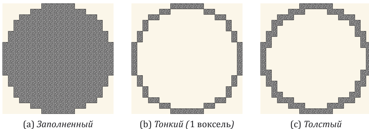
Рис. 2: Три режима рендеринга для одной и той же евклидовой окружности D = 20 . Режим Тонкий соответствует дискретной топологической границе ( \partial F ); режим Толстый добавляет диагональные блоки для закрытия отверстий под 45^\circ , что необходимо для герметичных построек (подводные купола из Стекла/Льда).
