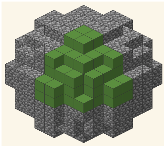
Рис. 7: Сфера D = 10 с положительным октантом (+x, +y, +z) , выделенным зелёным. При действии подгруппы \mathbb{Z}_2^3 \leq O_h (порядка 8, порождённой тремя координатными отражениями) этот октант определяет всю сферу — остальные семь областей получают последовательно /clone с mode:masked , применённой к октанту, построенному вручную.
