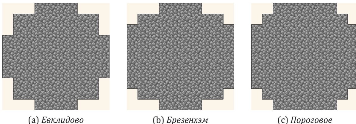
Рис. 1: Одна и та же окружность диаметра D = 10 при трёх различных критериях. Каждая фигура — это множество клеток, помеченных соответствующей версией неравенства d_x^2 + d_y^2 \leq 1 , отрендеренное текстурой cobblestone из Minecraft. Обратите внимание на различия в переходах между рядами, угловых клетках и кардинальных точках — три математически верных ответа при разных критериях.
