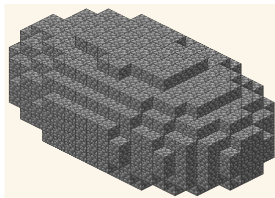
(b) Эллипсоид W = 20, H = 10, D = 12 .
