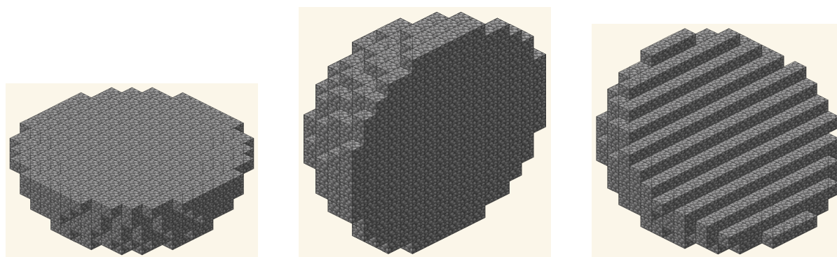
(a) Сечение Y 50% (купол)
