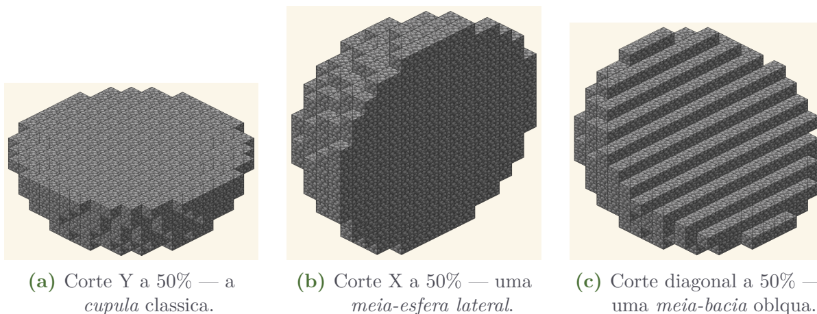
Figura 6: Tres cortes planares no mesmo elipsoide de diametro 16, todos preservando 50% do volume. Observe o padrao escalonado caracteristico do corte diagonal: ele expoe a hipotenusa que conecta os dois eixos. Cada corte e um plano de construcao Minecraft diferente: cupula de templo, meia-arena lateral, anfiteatro de fonte.
