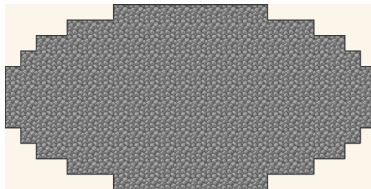
Figura 7: Elipse W = 24, H = 12 no Block Round. Note como as células ao longo do eixo maior são mais espaçadas que ao longo do eixo menor.
