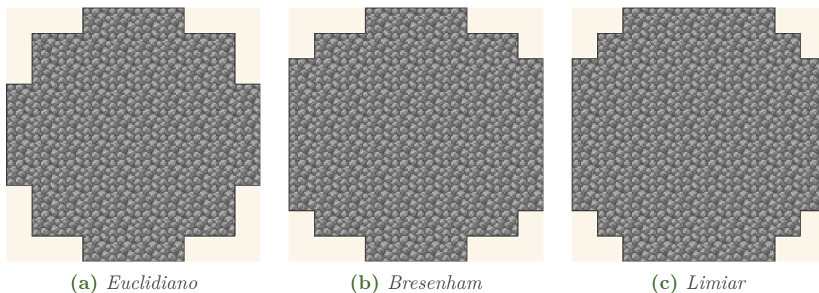
Figura 1: Mesma circunferência de diâmetro 10 sob três critérios de pertinência, renderizada com a textura cobblestone (pedregulho) do Minecraft. Observe como a célula de canto, a transição entre linhas e os pontos cardiais variam de uma para outra — são três respostas matematicamente corretas sob critérios distintos, e três planos de construção diferentes em Minecraft .
