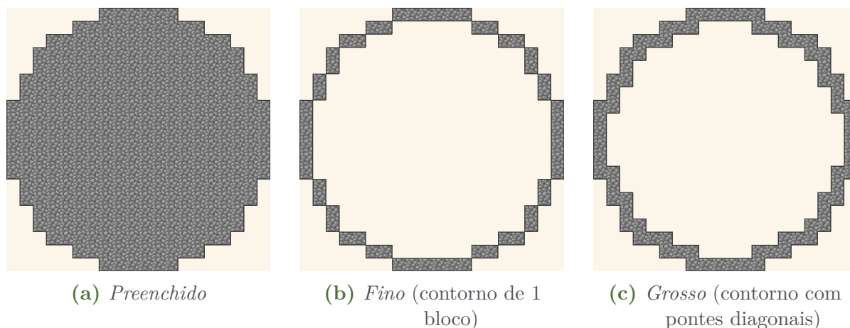
Figura 2: Os tres modos de renderizacao para a mesma circunferencia euclidiana de diametro 20. O modo Fino corresponde ao bordo discreto topologico; o modo Grosso adiciona blocos nas diagonais para evitar buracos a 45^\circ — exatamente o problema que aparece em uma cupula de Vidro subaquatica do Minecraft, onde uma fenda diagonal deixa a agua entrar.
