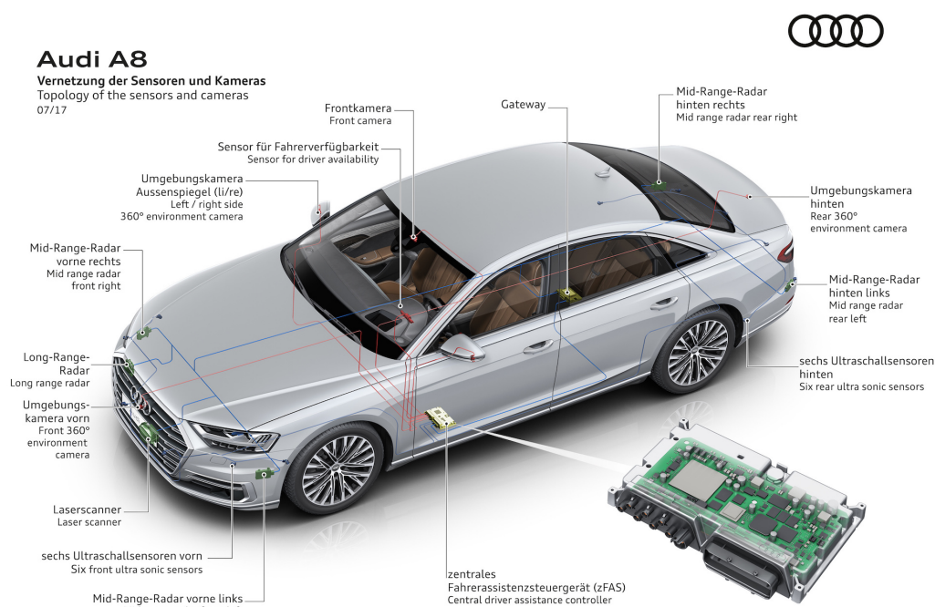
Figura 1 – Sensores e Câmeras do Audi A8
