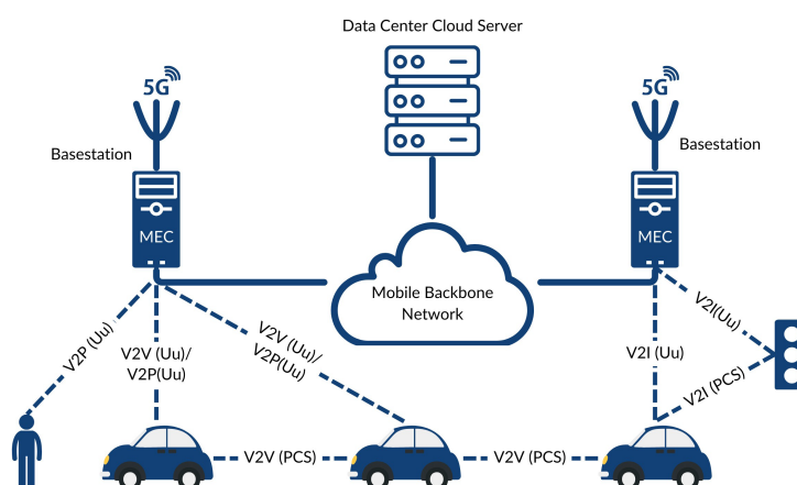
Figura 8 – Ilustração de um sistema C-V2X
