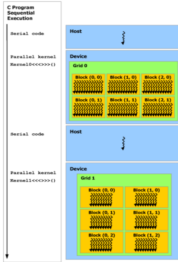
Figura 3 – Execução de um programa feito em CUDA.
