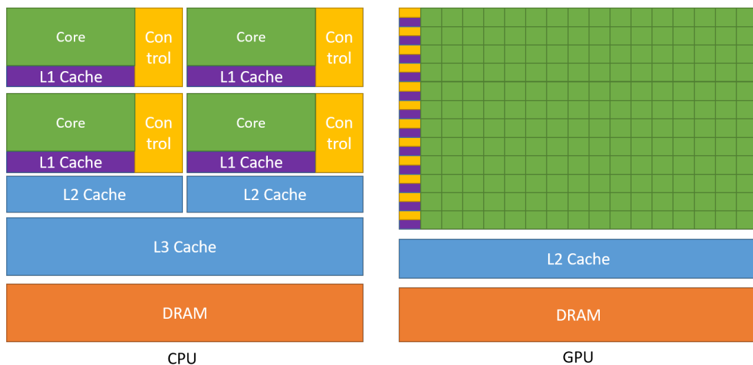
Figura 2 – Arquitetura de uma CPU e de uma GPU.
