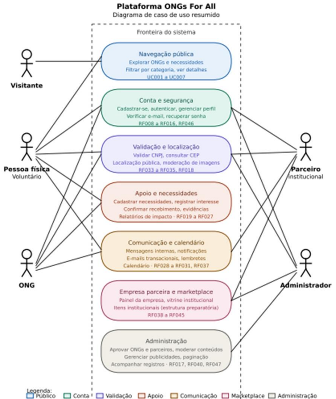
Figura 1 - Diagrama de caso de uso resumido da plataforma ONGs For All
