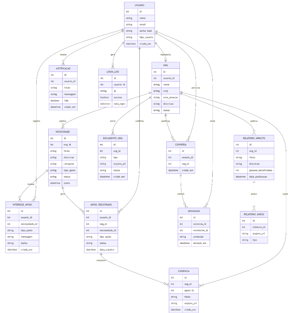
Figura 10 - Modelo Entidade-Relacionamento conceitual da plataforma ONGs For All
