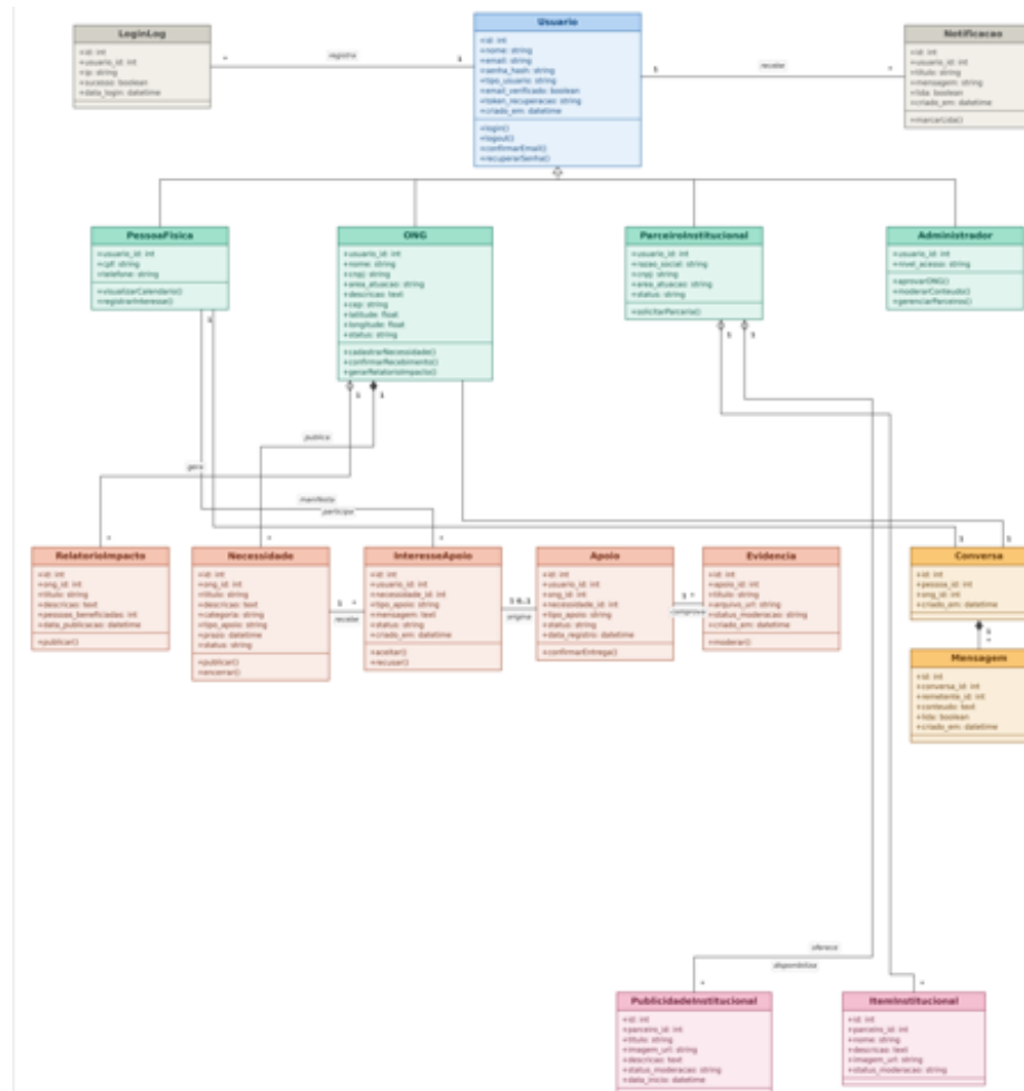
Figura 2 - Diagrama de Classes da plataforma ONGs For All
