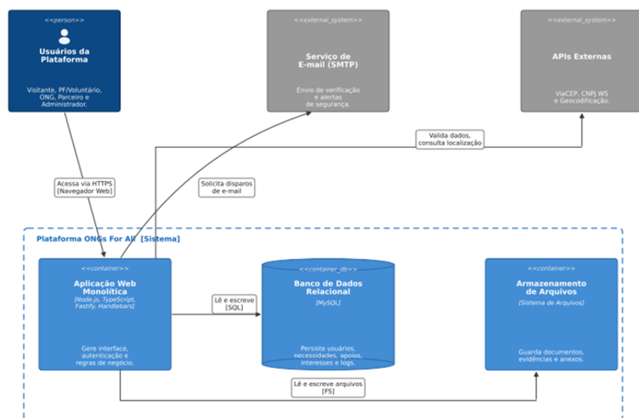
Figura 13 - Diagrama de Contêineres da plataforma ONGs For All
