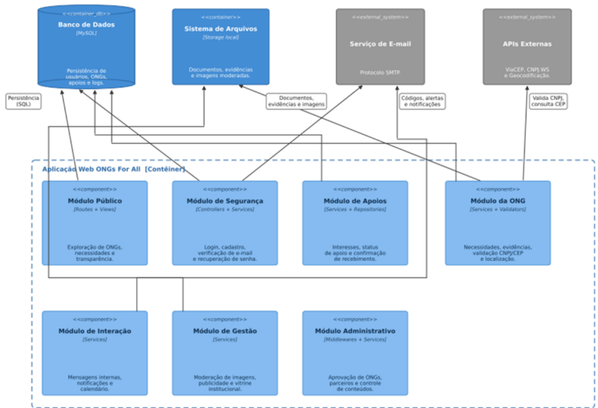
Figura 14 - Diagrama de Componentes da aplicação ONGs For All
