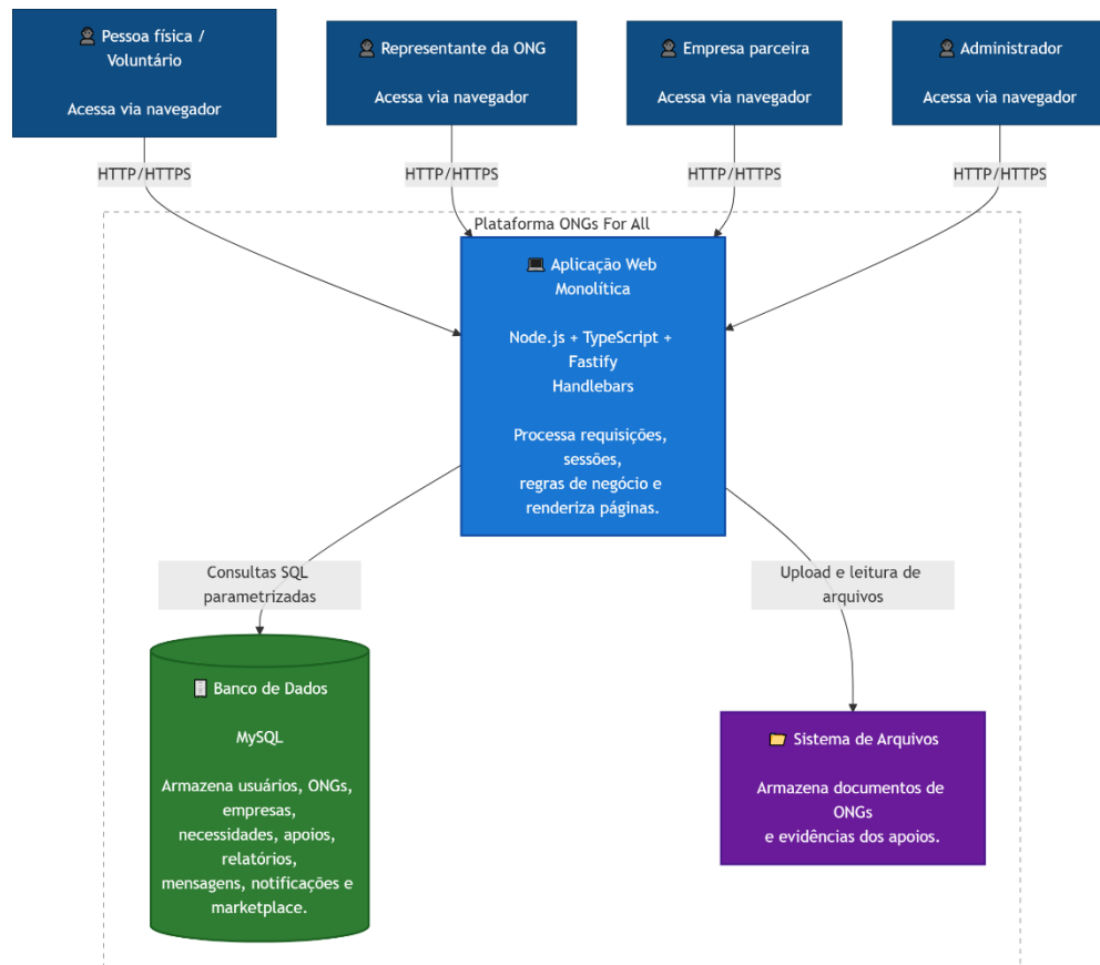
Figura 13 - Diagrama de Contêineres da plataforma ONGs For All
