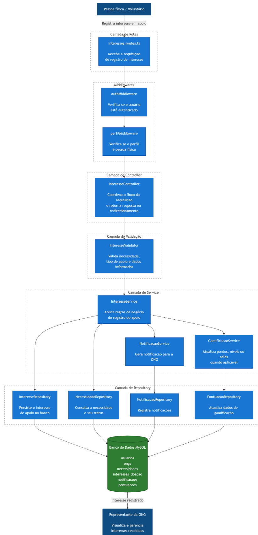
Figura 15 - Diagrama de Código do fluxo de registro de interesse em apoio
