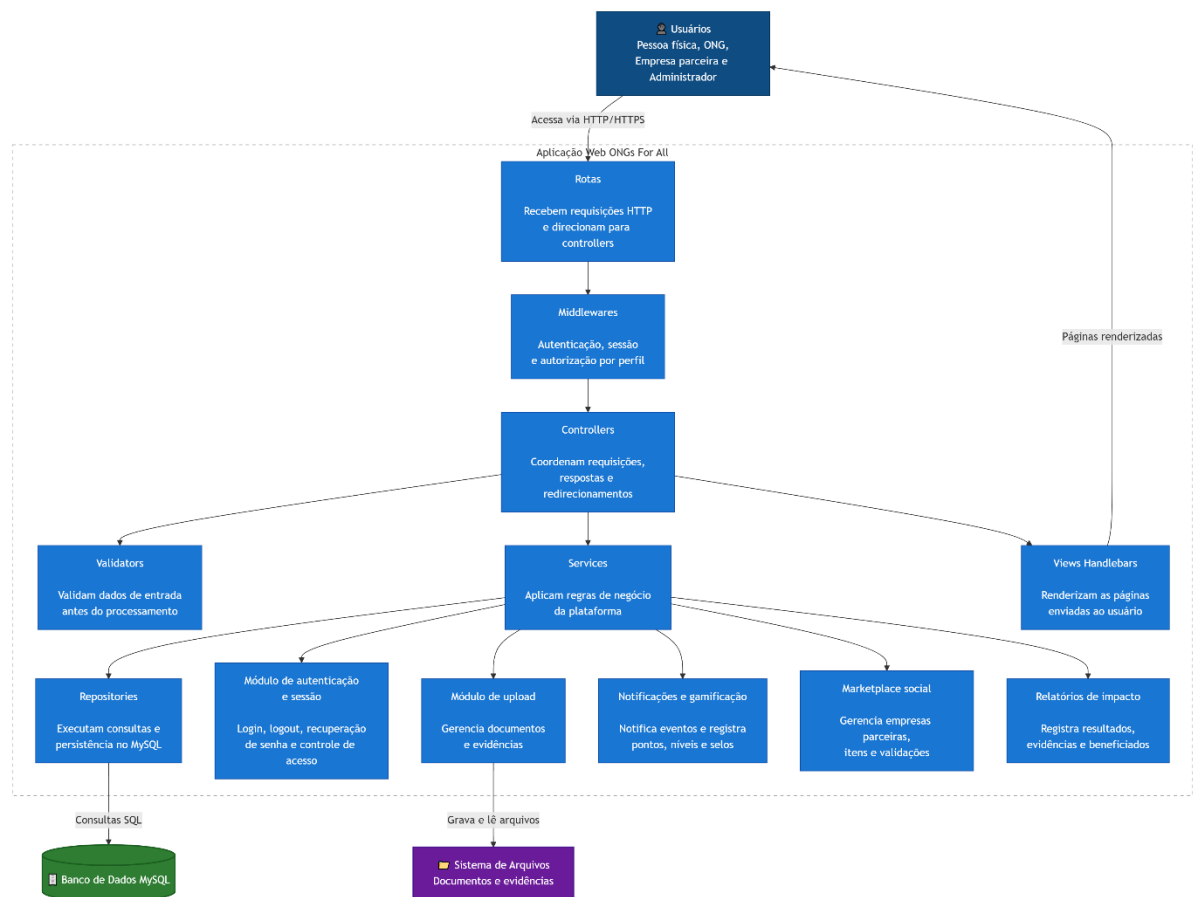
Figura 14 - Diagrama de Componentes da aplicação ONGs For All
