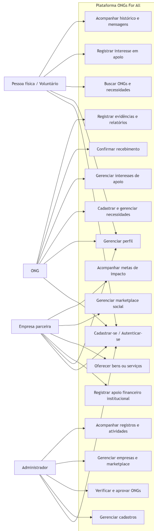
Figura 1 - Diagrama de caso de uso resumido da plataforma ONGs For All
