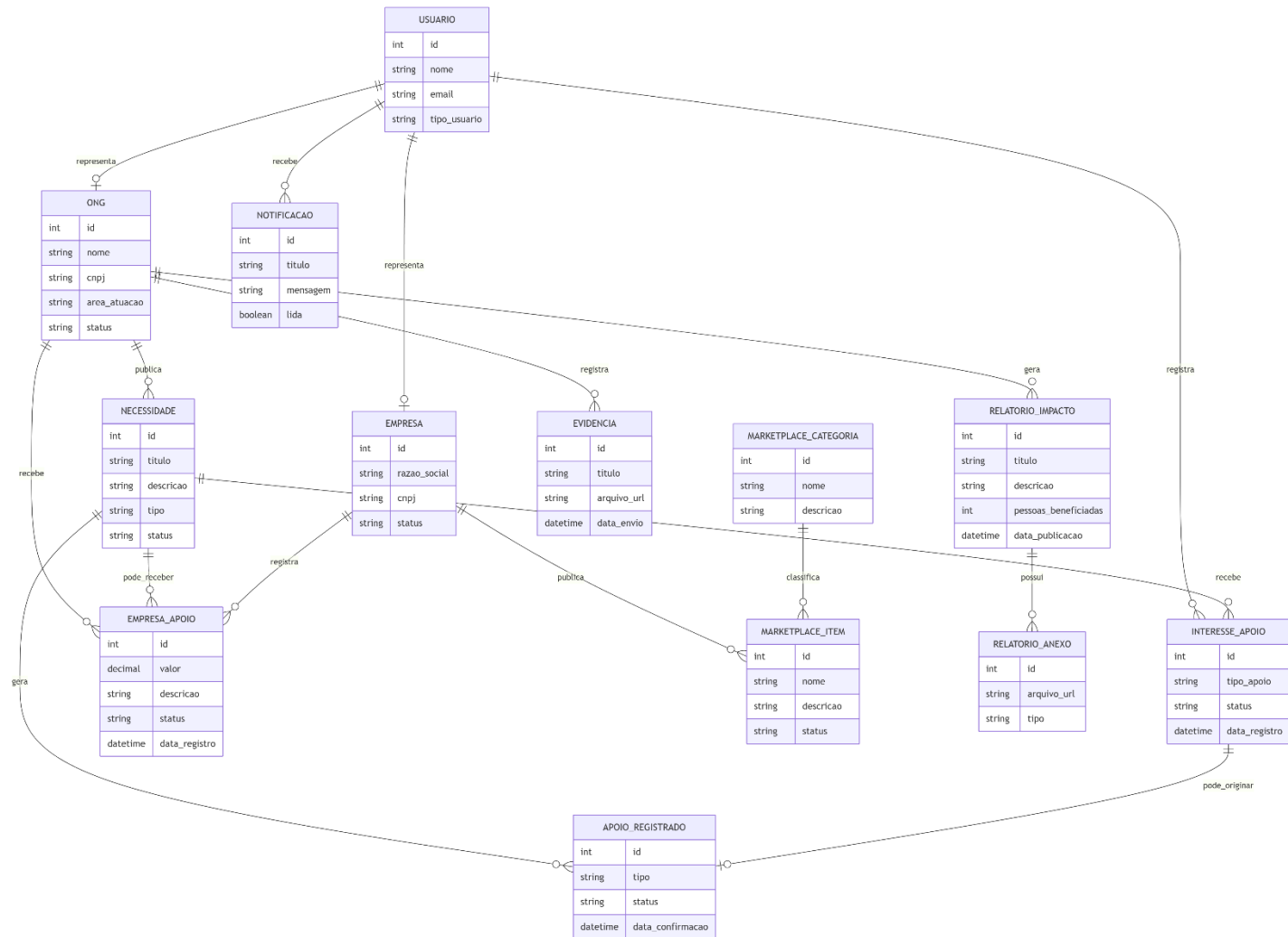
Figura 10 - Modelo Entidade-Relacionamento conceitual da plataforma ONGs For All
