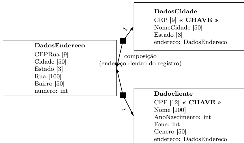
Figura 2: Estruturas de dados e relações de composição entre endereço, cidade e cliente.
