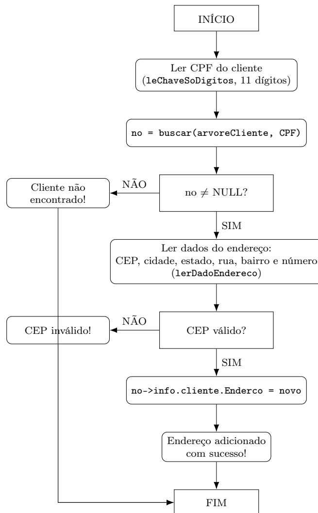
Figura 4: Fluxograma do cadastro do endereço de um cliente.
