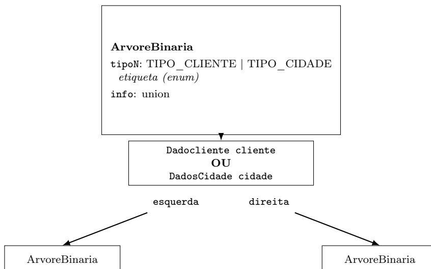
Figura 3: Nó genérico da árvore binária com união, etiqueta de tipo e ponteiros para os filhos.
