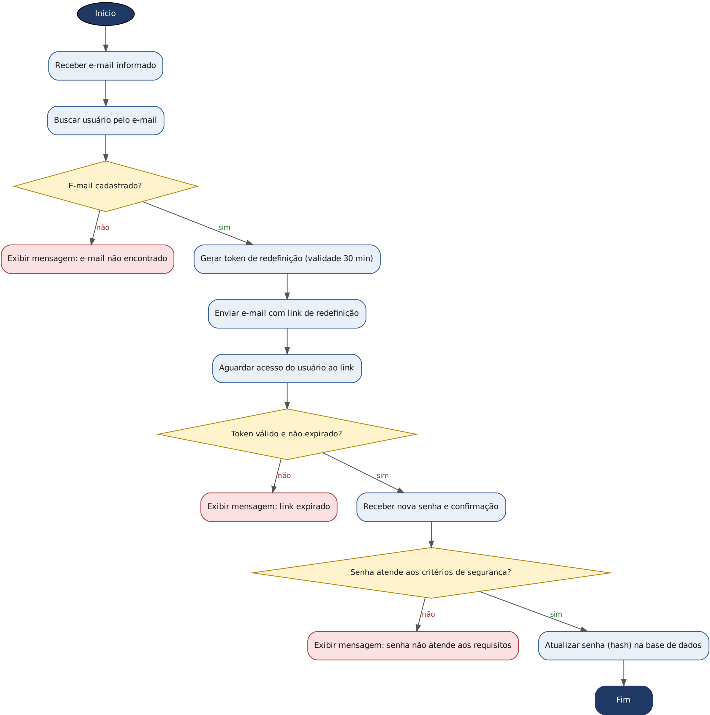
Usuario.recuperarSenha(email): void — Diagrama de Atividades (nível de algoritmo)
