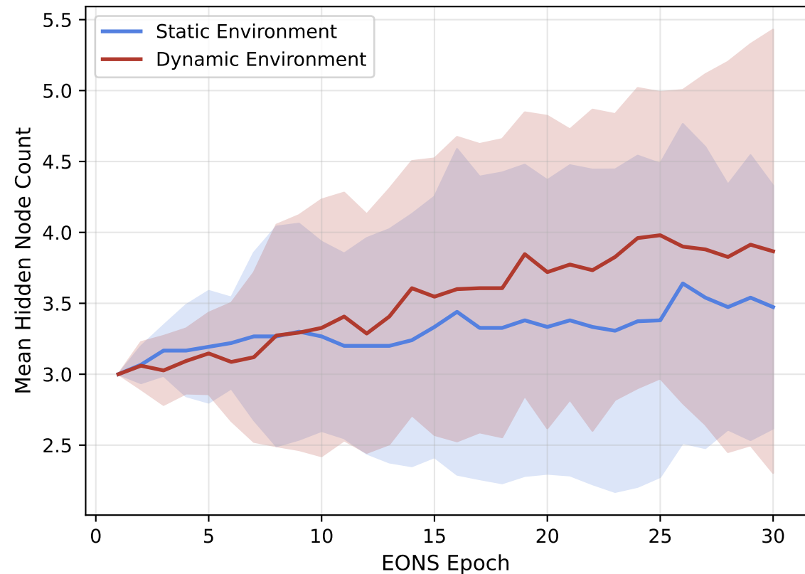
Mean Hidden Nodes per Population
