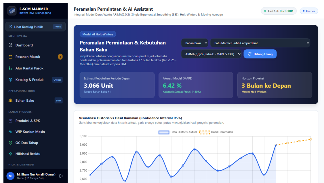
Gambar 11.1: Grafik Peramalan Permintaan AI Menggunakan Model Terbaik ARIMA(2,0,2)
