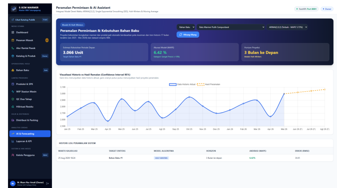
Gambar 11.1: Grafik Peramalan Permintaan AI Menggunakan Model Terbaik ARIMA(2,0,2)
