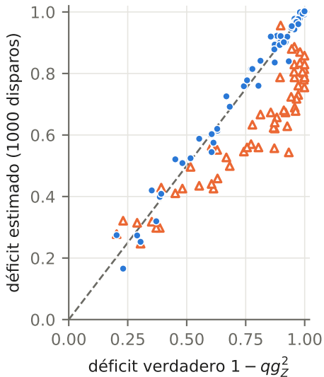
(a) T1 igual, 6 qubits, peso 2, profundidad 24
