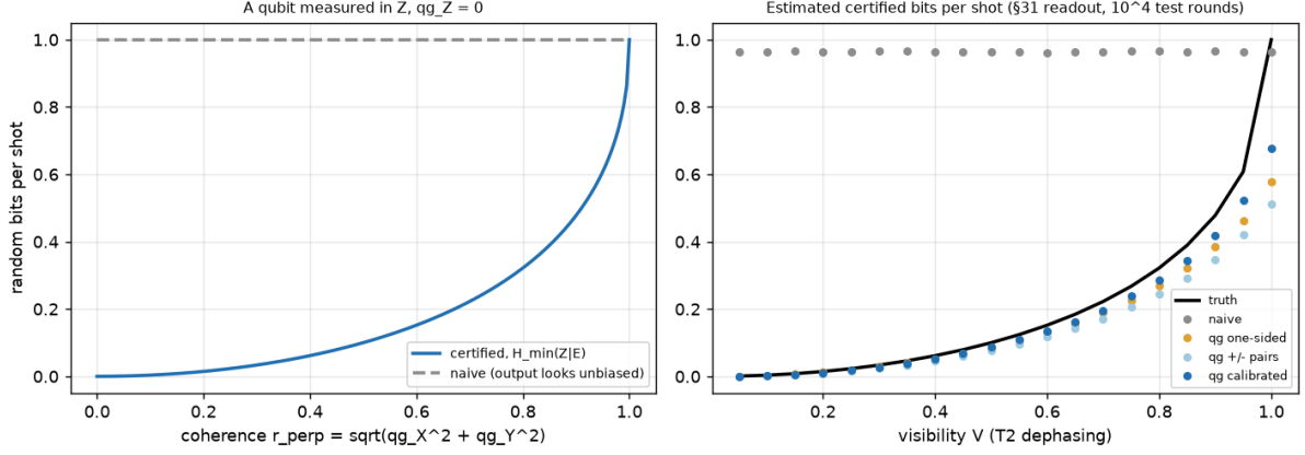
Figura 3: Izquierda: bits certificados por disparo según la coherencia r_{\perp} con qg_Z = 0 , frente a la lectura ingenua. Derecha: estimaciones según la visibilidad V .
