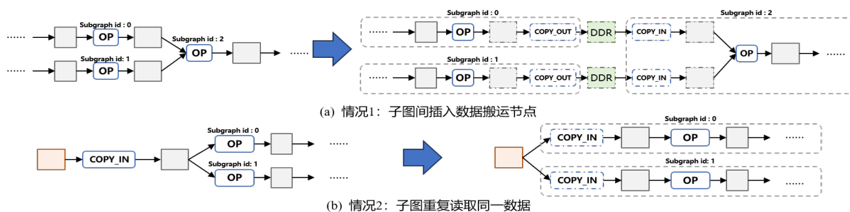
图 2 切图后数据搬运节点插入规则
