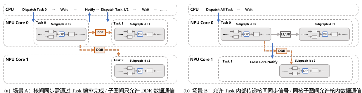
图 3 两种场景下子图间通信方式对比
