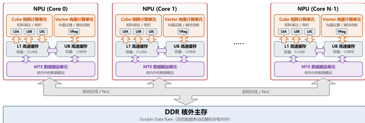
图 4 多核 NPU 平台硬件架构
