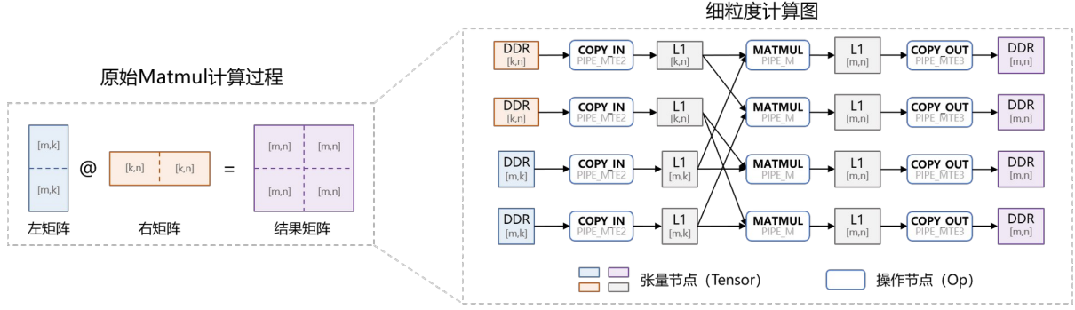
图 1 矩阵乘法的示例计算图
