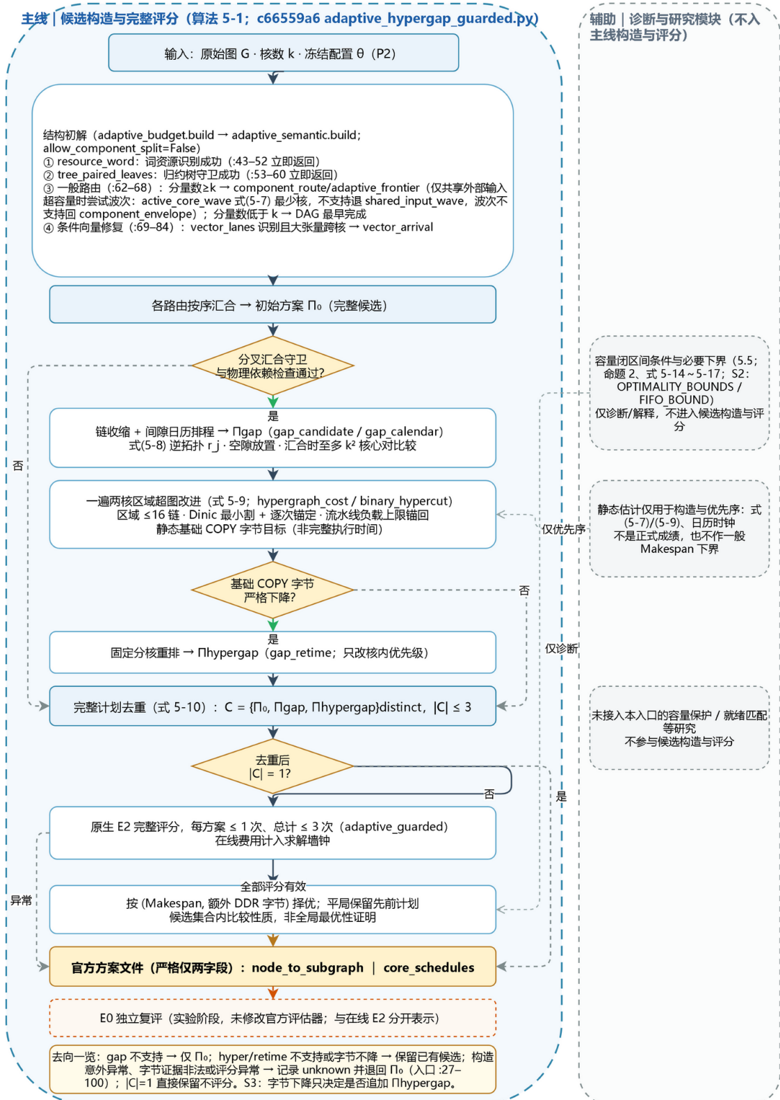
图 5.1 P2 张量通信优化技术路线: 结构初解 \Pi_0 (含式 (5-7) 活跃核选择与条件向量通路修复) \rightarrow 分叉汇合守卫 \rightarrow \Pi_{gap} \rightarrow 两核区域超图改进 \rightarrow 字节判定 \rightarrow \Pi_{hypergap} \rightarrow 去重 ( |C| \leq 3 ) \rightarrow E2 评分择优 (异常退回 \Pi_0 ) \rightarrow 两字段方案 \rightarrow E0 复评; 侧栏为诊断与研究模块。结构与方法流程图, 不声称实测加速或零 spill。
