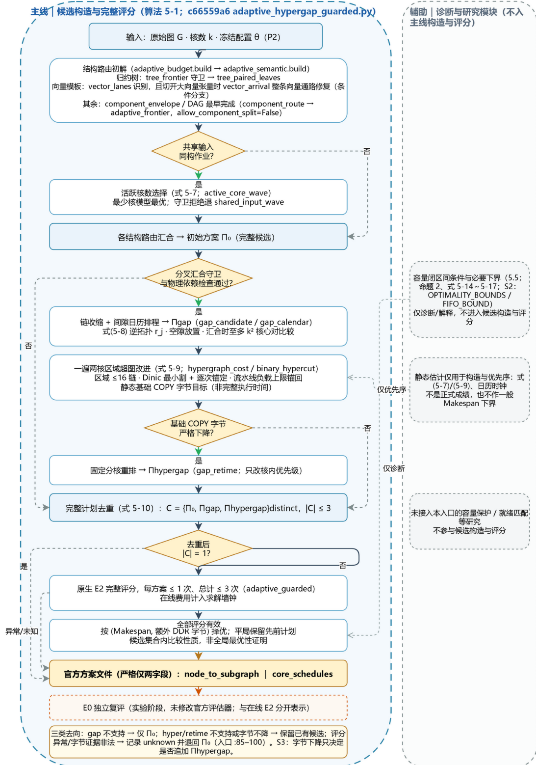
图 5.1 P2 张量通信优化技术路线: 结构路由初解 \Pi_0 (含式 (5-7) 活跃核选择与条件向量通路修复) \rightarrow 分叉汇合守卫 \rightarrow \Pi_{gap} \rightarrow 两核区域超图改进 \rightarrow 字节判定 \rightarrow \Pi_{hypergap} \rightarrow 去重 ( |C| \leq 3 ) \rightarrow E2 评分择优 (异常退回 \Pi_0 ) \rightarrow 两字段方案 \rightarrow E0 复评; 侧栏为诊断与研究模块。
