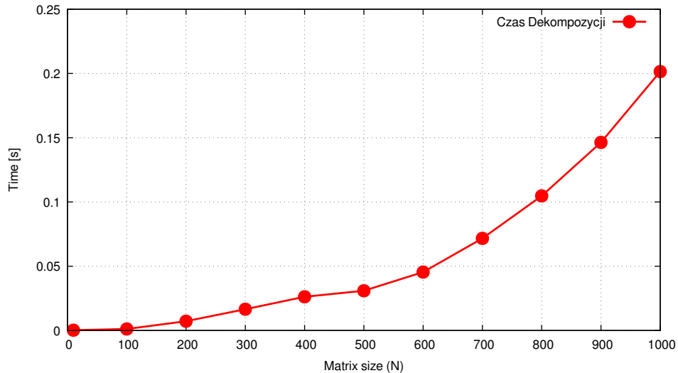
Złożoność czasowa dekompozycji LU ( O(N^3) )
