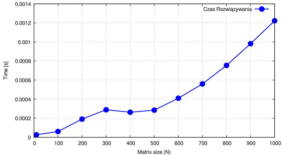
Złożoność czasowa rozwiązywania układu ( O(N^2) )
