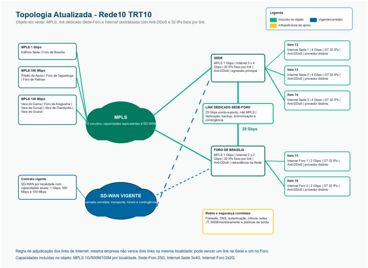
Figura 1 - Arquitetura proposta MPLS, SD-WAN, link dedicado Sede-Foro e Internet centralizada
