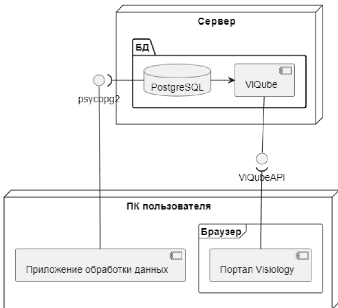
Рисунок 7 - Диаграмма развертывания
