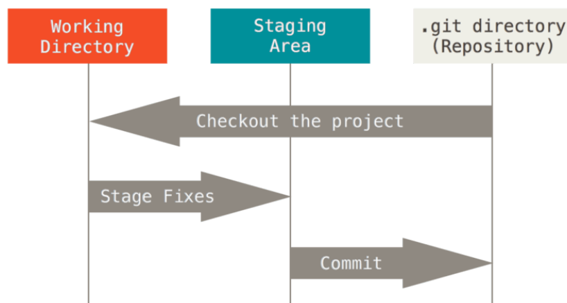
Figura 3.1: Tipico workflow git per effettuare il versioning di file
