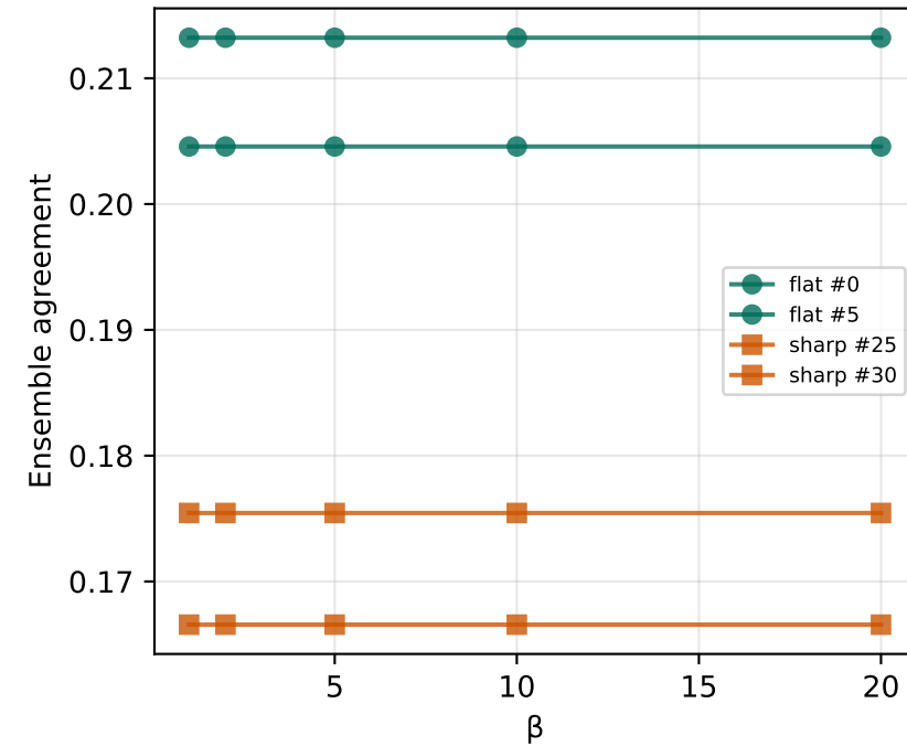
(d) Ensemble agreement invariant
